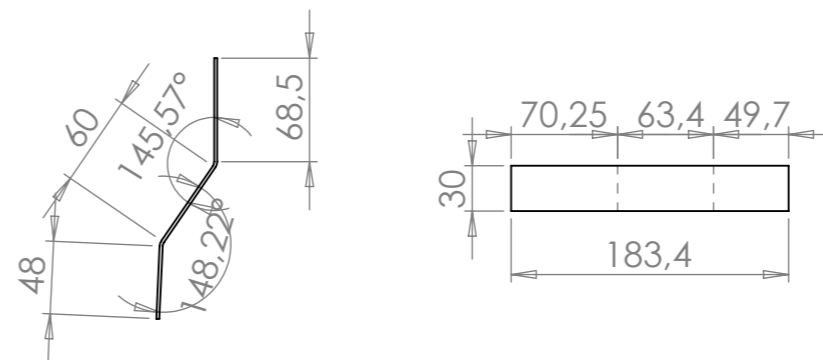
Bockad plåt för infästning mot pappeskorgen.
